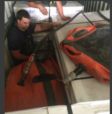
Load Shift Inside Van Trailer
